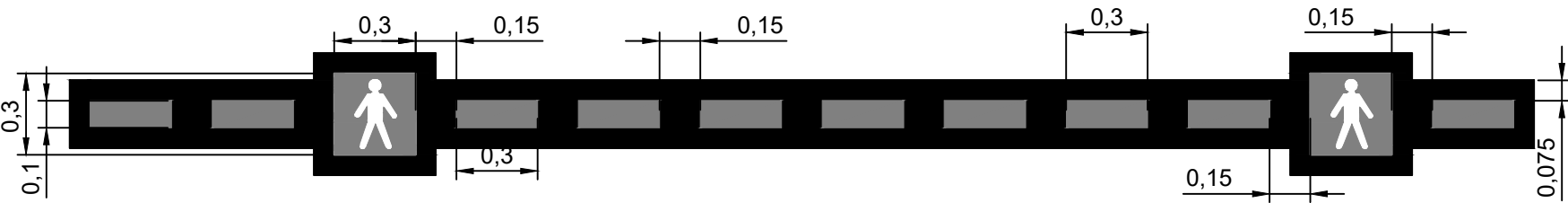
SEÑAL DE SENDA PEATONAL EN PLATAFORMA
