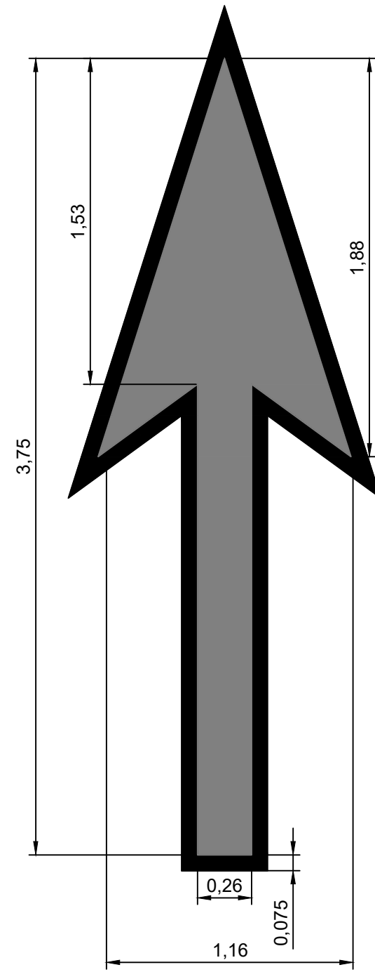
SEÑAL INDICADORA SENTIDO DE CIRCULACIÓN
