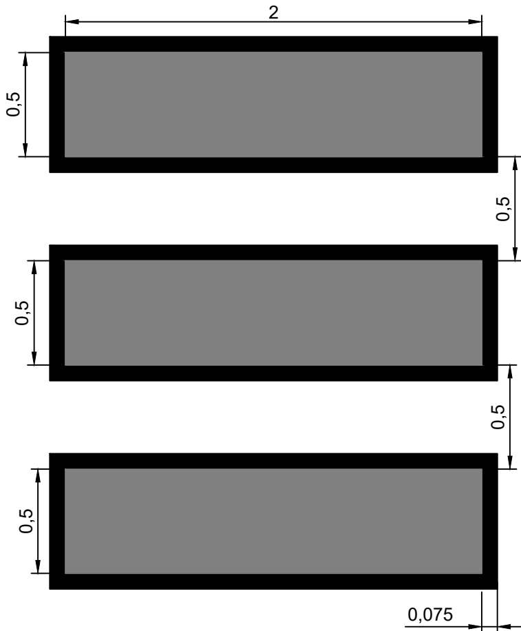
SEÑAL DE SENDA PEATONAL EN CALLE VEHICULAR
