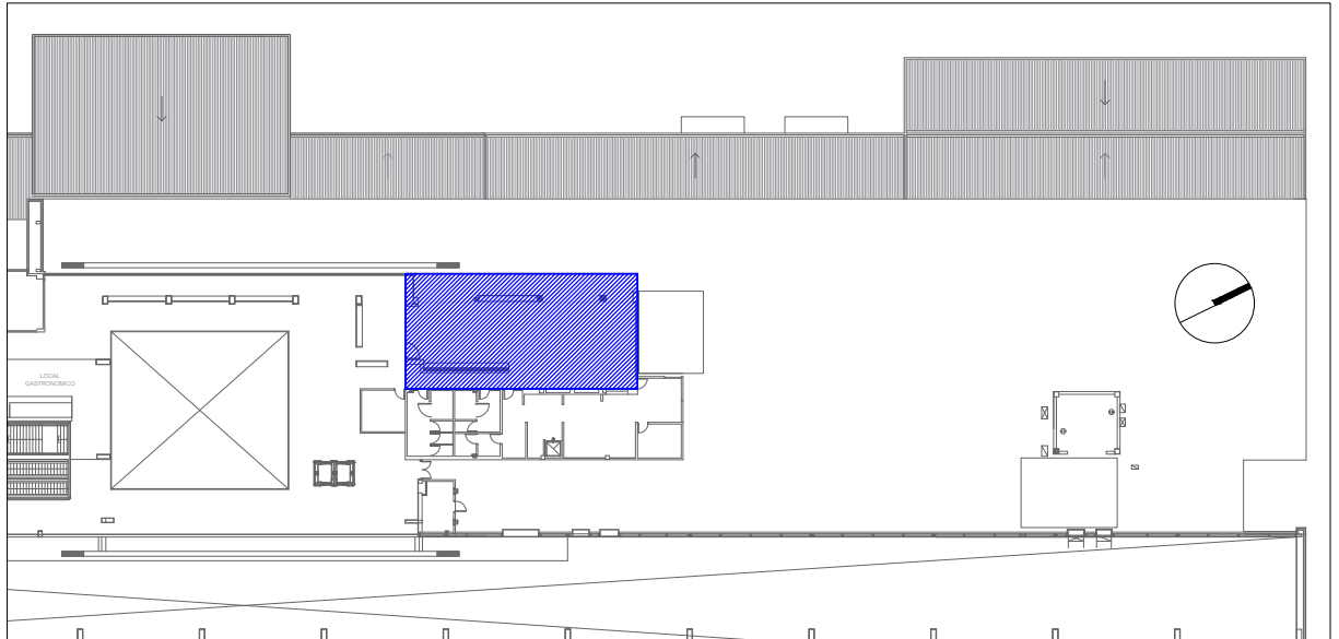
UBICACIÓN DEL LOCAL - PA TERMINAL DE PASAJEROS
