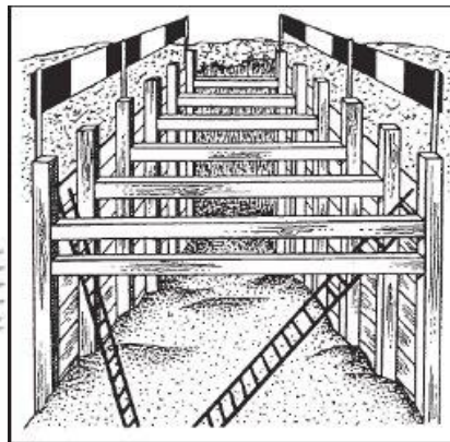
Entibado
