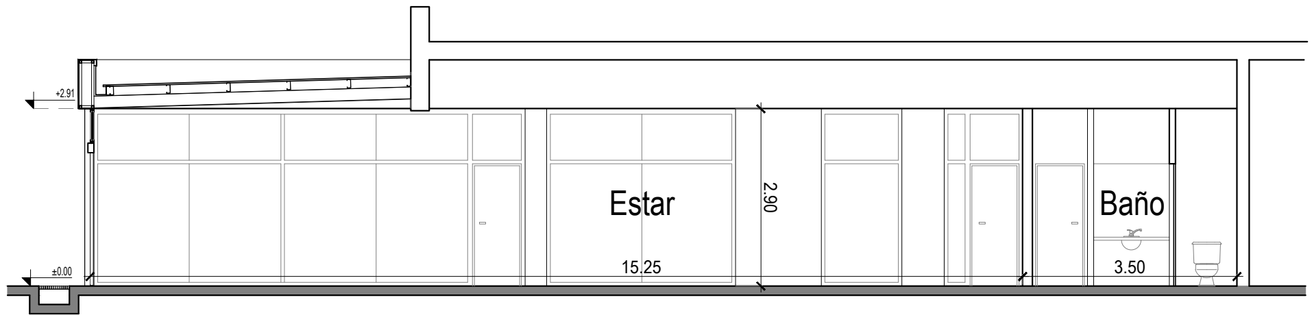
Corte longitudinal- Sala Vip internacional
