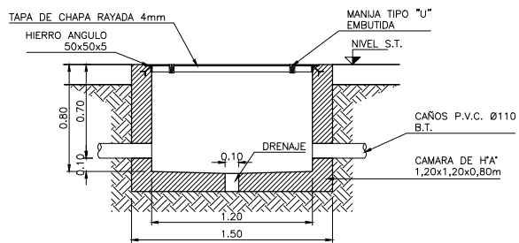
CAMARA TIPO E01 CORTE 1-1 ESC. 1:20
