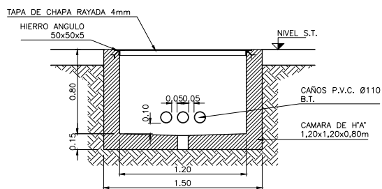
CAMARA TIPO E01 CORTE 2-2 ESC. 1:20
