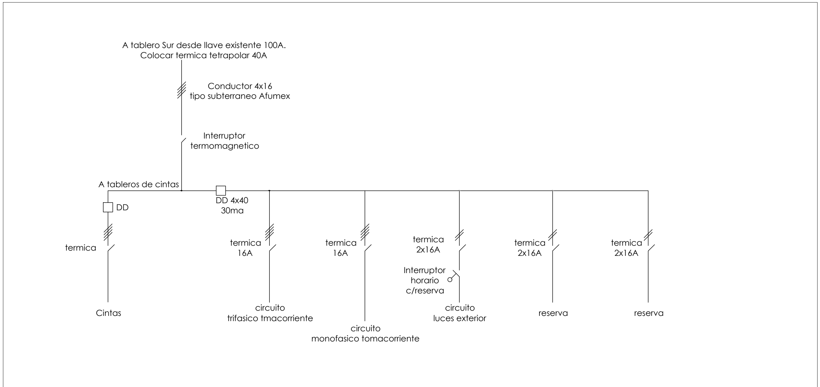
Esquema unifilar- tablero n°1
