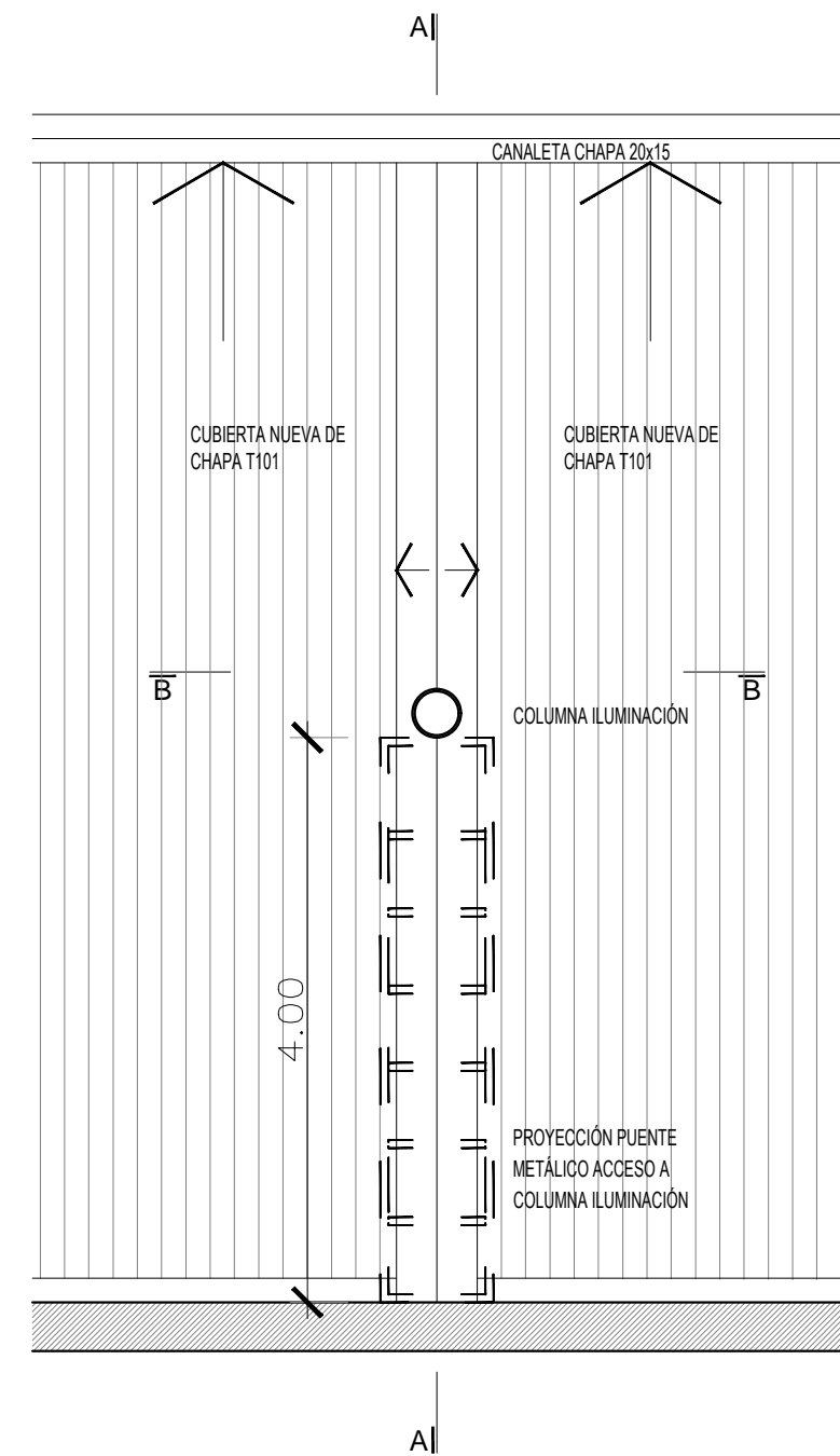
Planta Techos- sector aislación columna de iluminación esc. 1:50
