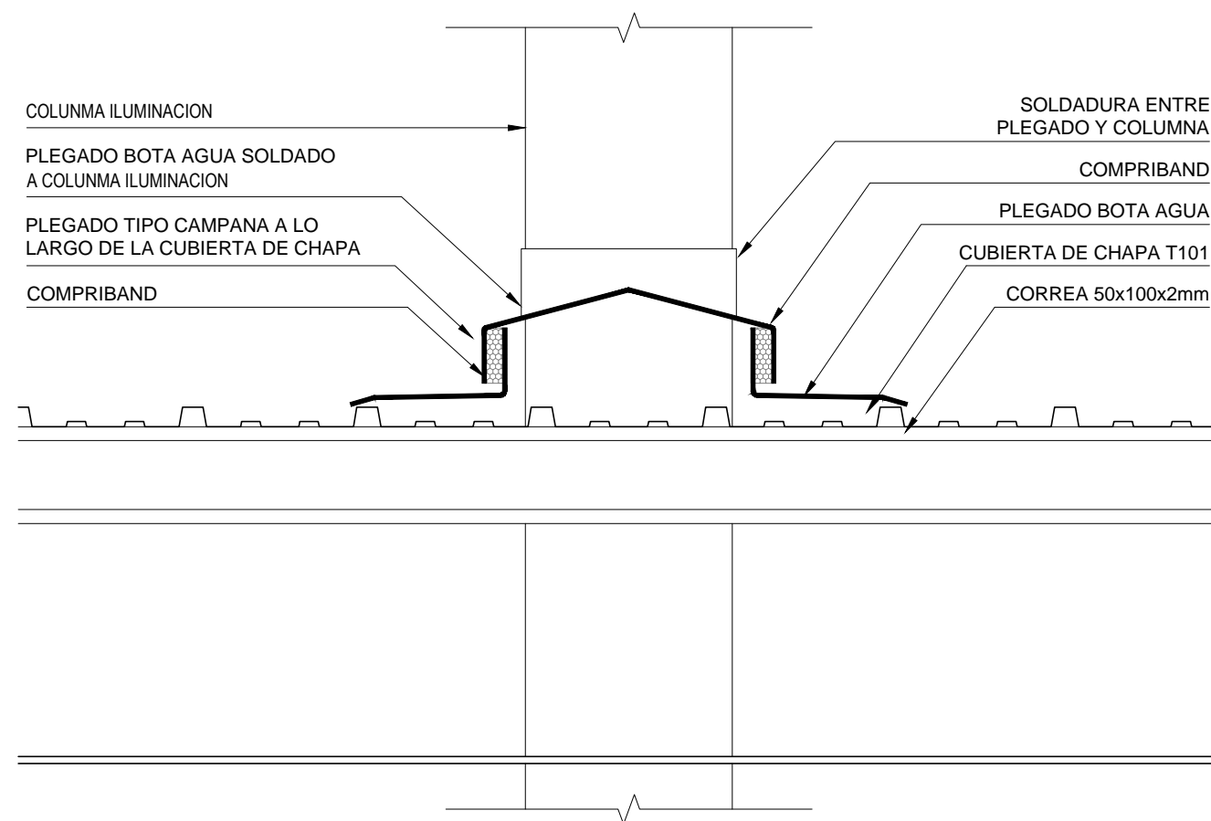
Detalle B-B esc. 1:10
