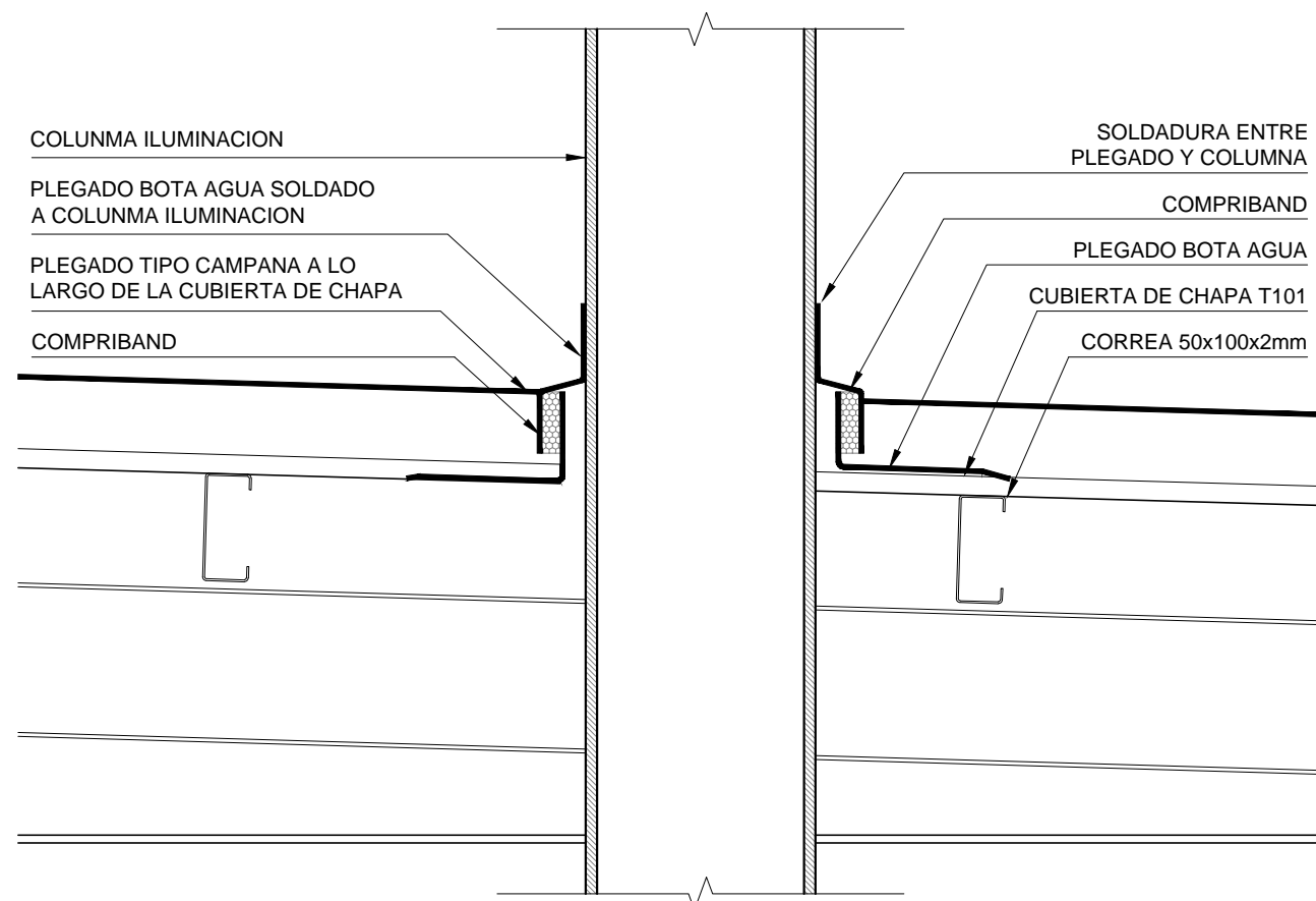
Detalle A-A esc. 1:10
